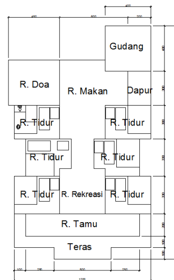
Denah Rumah tinggal Pengelola
